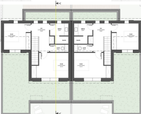
Plan du R+1
